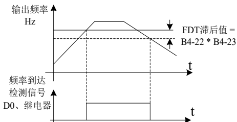
图 5-14 FDT 电平示意图
