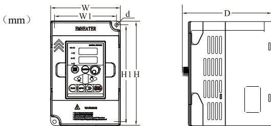
图 2-3 ACH800 单相/三相 0.75~2.2kW 壁挂安装尺寸图
