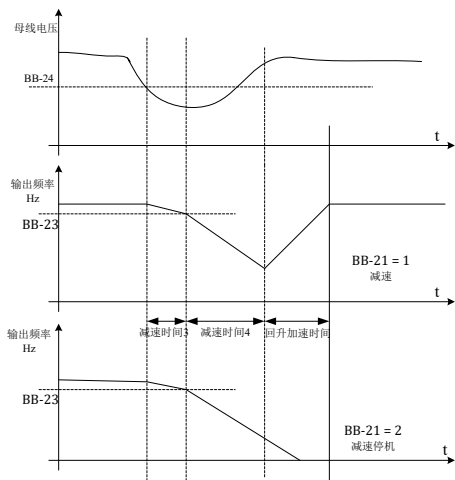
图 5-24 瞬时停电动作示意图
