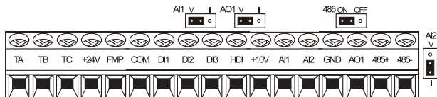
图 3-12 ACH800 单相/三相 0.75 kW ~ 2.2kW 控制回路端子图
