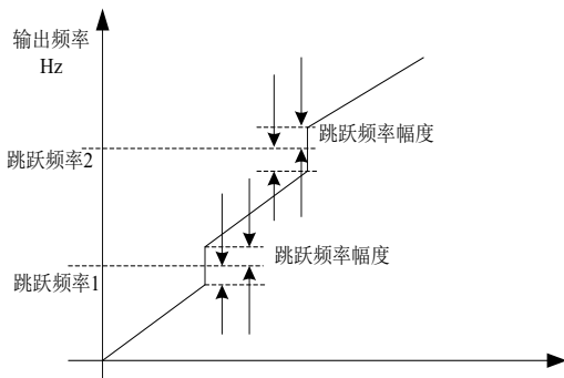
图 5-7 加减速过程中跳跃频率有效示意图
