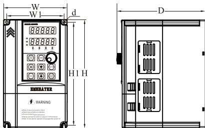
图 2-40 三相 4~22kW 壁挂安装尺寸图
