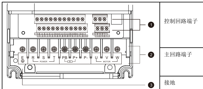
图 3-7 ACH800 系列端子布局图示
