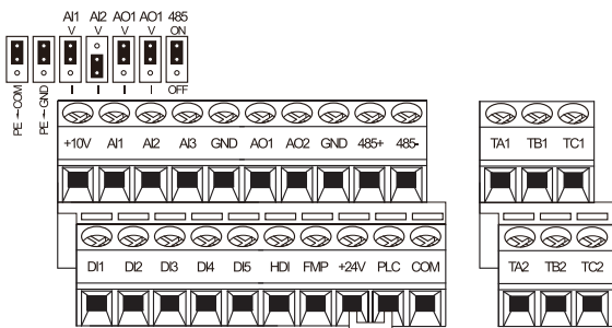
图 3-13 ACH800 三相 4kW 以上控制回路端子图
