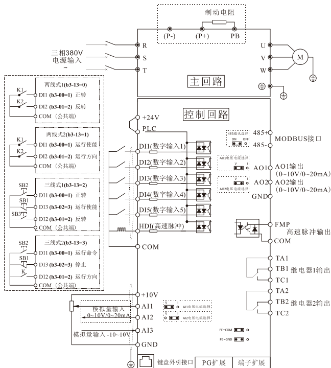
3-11 ACH800控制回路及主回路接线图
