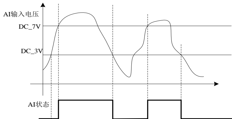
图 5-22 AI 端子有效状态判断
