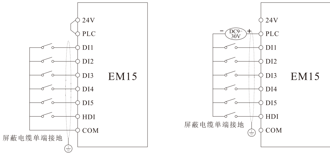
图 3-14 两种不同模式下数字输入端子接线图
