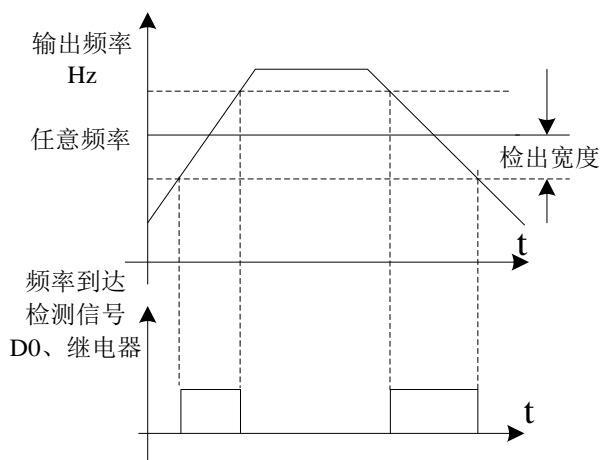
图 5-16 任意到达频率检测示意图
