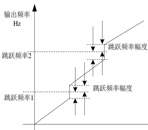
图 5-7 加减速过程中跳跃频率有效示意图
