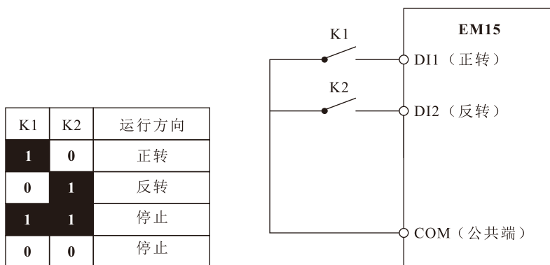
图 5-10 两线式模式 1
