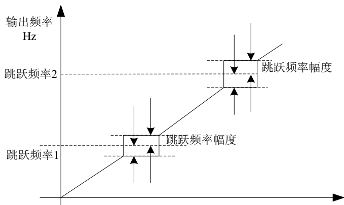
图 5-6 跳跃频率示意图
