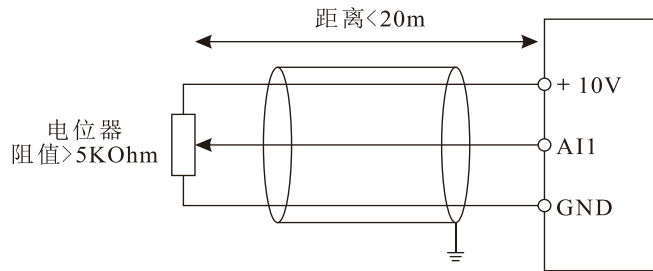
图 3-15 模拟量输入端子接线方式
