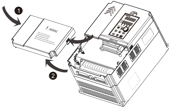
图3-5塑壳机箱下面板的拆卸
