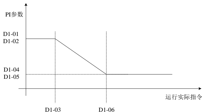
图 5-29 PI 参数示意图
