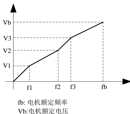
图 5-31 多点 V/F 曲线设定示意图
