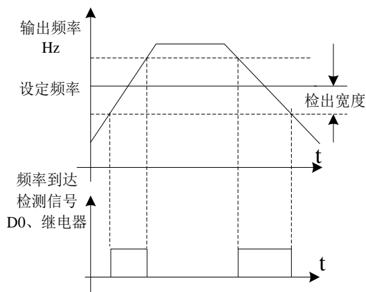
图 5-15 频率到达检出幅值示意图
