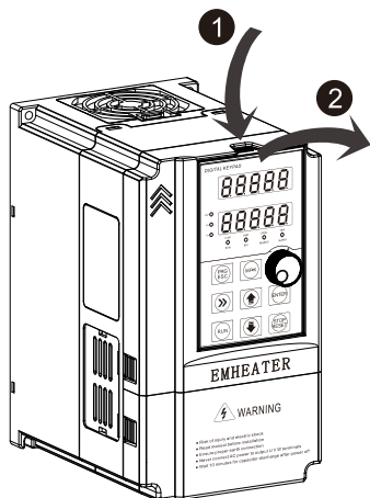
图 3-3 操作面板（键盘）的拆卸图
