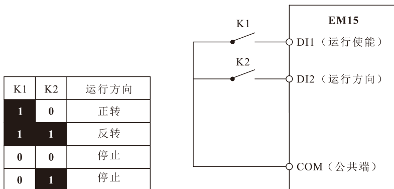
图 5-11 两线式模式 2
