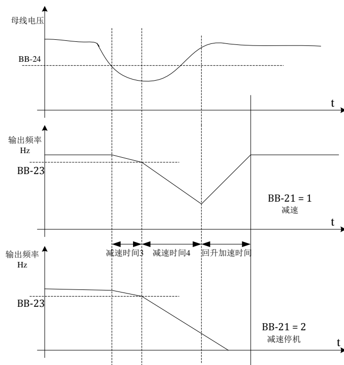
图 5-24 瞬时停电动作示意图
