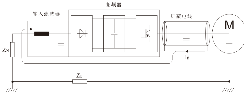
图 3-9 防传导辐射干扰接线示意图
